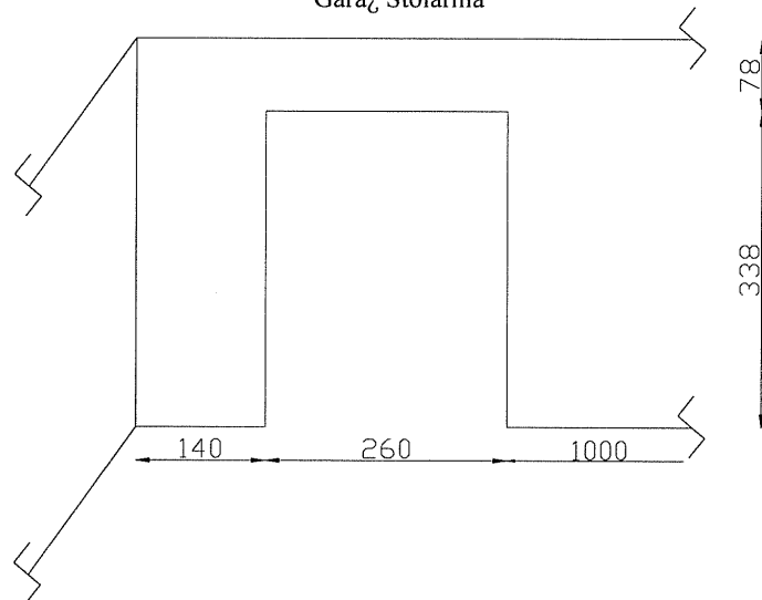
WIDOK OD WEWNĘ TRZ Garaż Stalarnia
