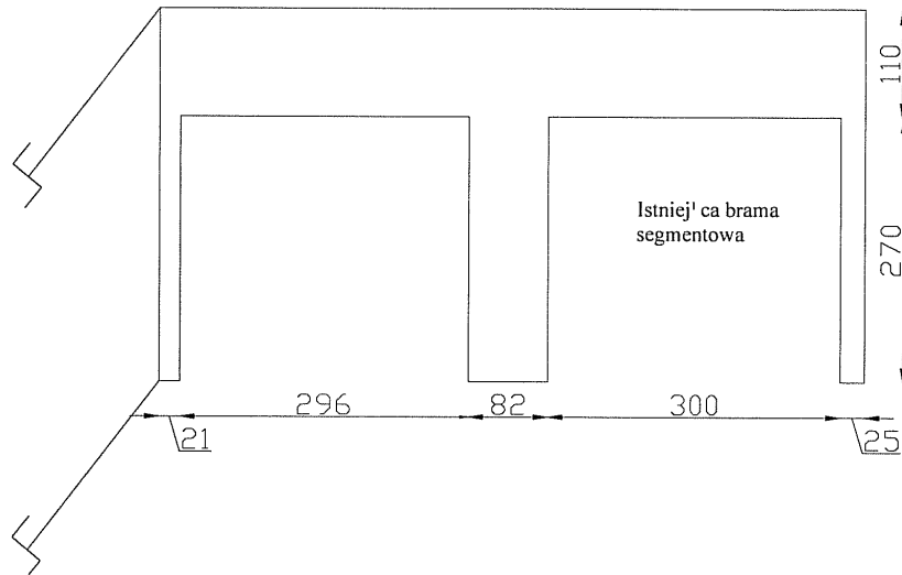
WIDOK OD WEWNĘ TRZ Garaż na UW Prosta
